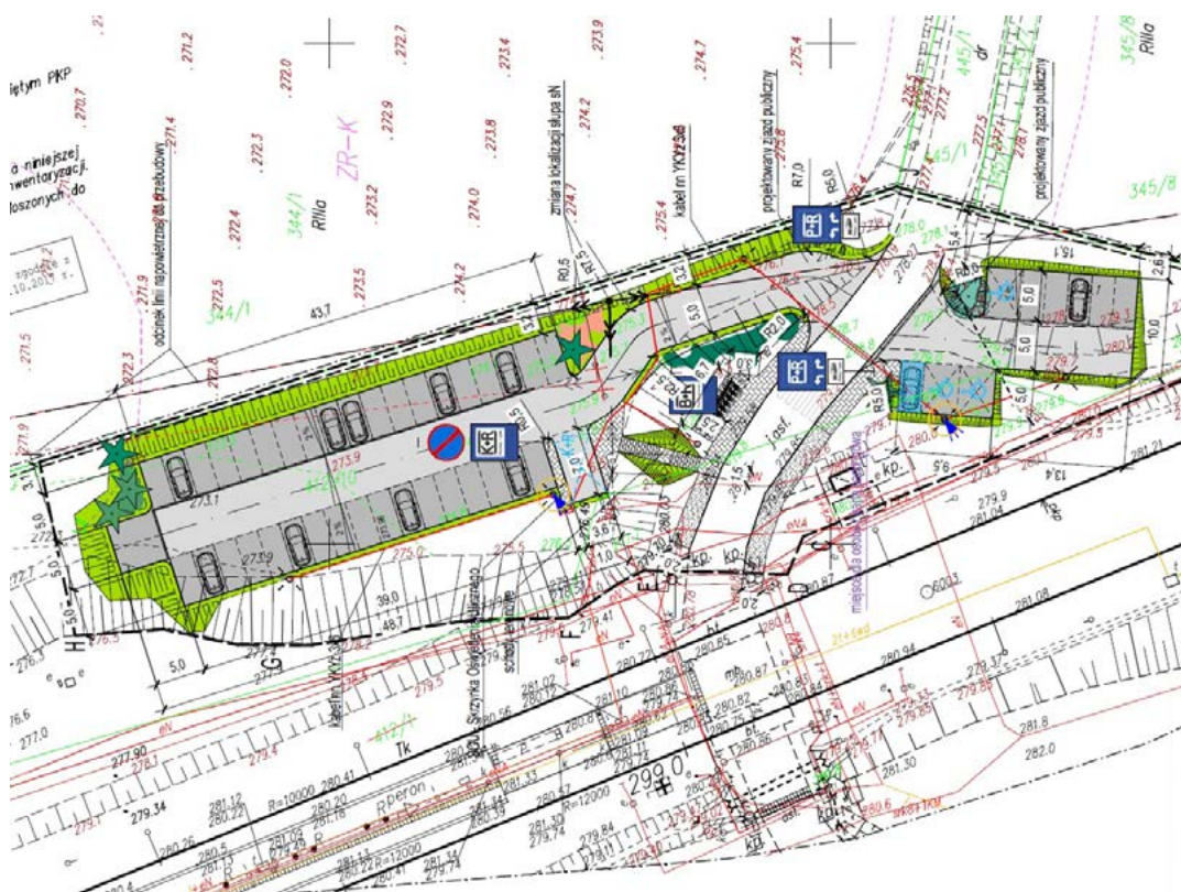
Parking w Goszczy – mapa do celów projektowych
